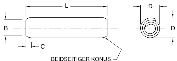
BEIDSEITIGER KONUS
